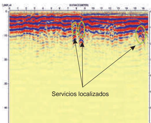
Ejemplo de radargrama donde se detectan servicios enterrados.
