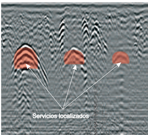
Ejemplo de radargrama donde se detectan servicios enterrados.
